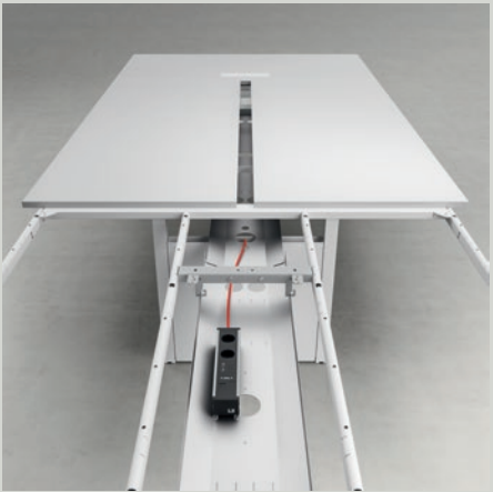
Dettaglio canale passacavi Detail of sheet metal cable duct
