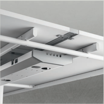
Canale passacavi in lamiera per bench - ispezionabile Sheet metal cable duct for bench - accessible
