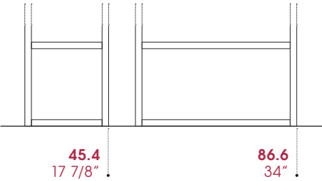
Larghezza moduli 45.4 - 86.6 cm / Width modules 17 7/8" - 34"
