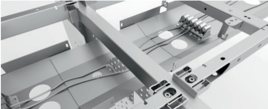
Canale passacavi ispezionabile doppio in lamiera / Inspectable equippable wire management double, in metal sheet
