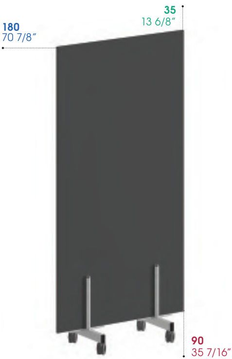
Partizione in melaminico sp. 1,8 cm con base su ruote / Melamine partitions 3/8" thick, with base on castors
