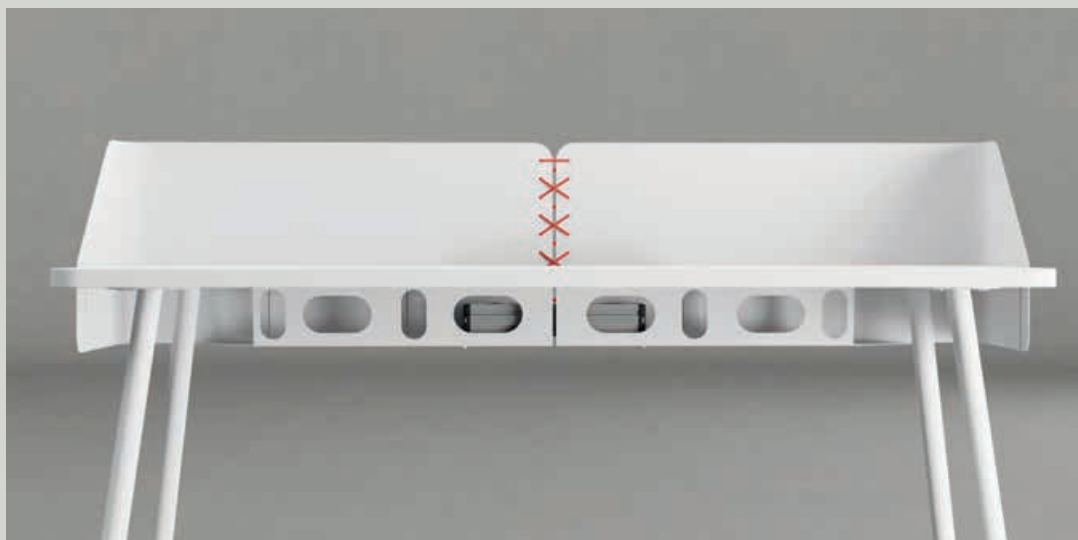
Canale passacavi in lamiera - ispezionabile Sheet metal cable duct - accessible
