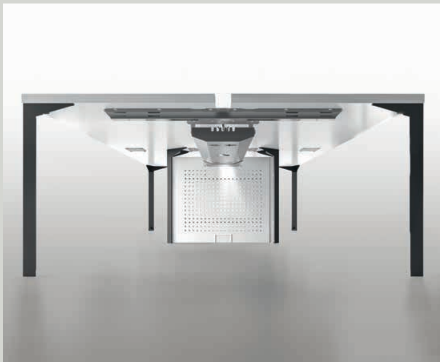
Dettaglio canale passacavi in lamiera per bench - ispezionabile Detail of sheet metal cable duct for bench - accessible
